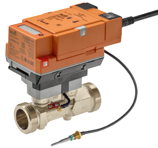
Fig. 48: Thermal energy meter from Belimo.
