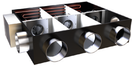
Fig. 80: Fan coil
