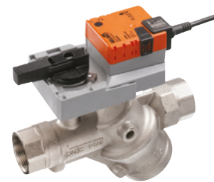
Fig. 2: PICCV
